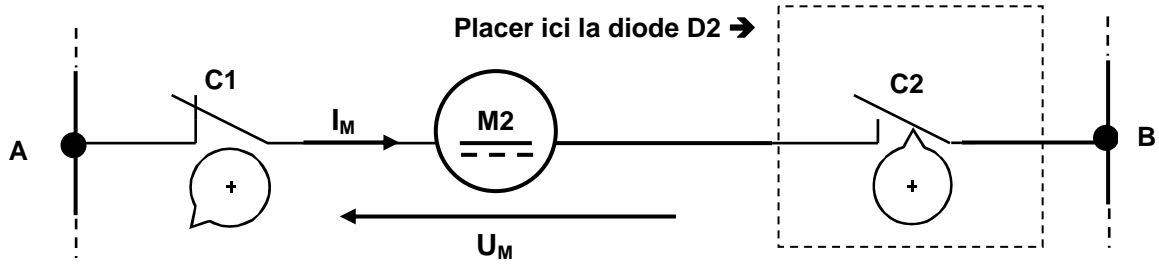
Figure 20 : NOTA : Les grandeurs U_M et I_M indiquées correspondent au redémarrage du moteur.
